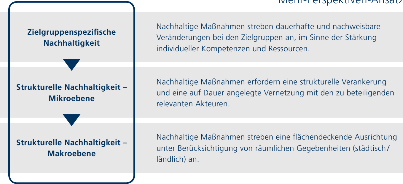
Abbildung 17: Mehr-Perspektiven-Ansatz
